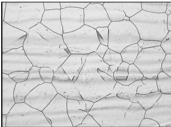
Microstructure x 275 / longitudinal
